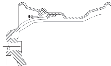
Außenliegendes Ventil (ALV)
