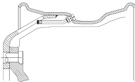
Innenliegendes Ventil (ILV)
